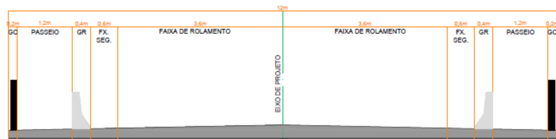
Fig. 5: Seção-tipo exigida
