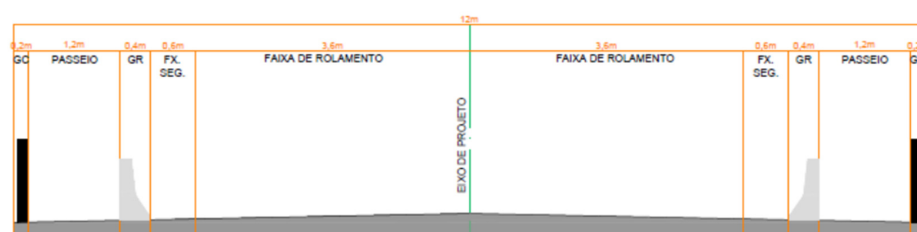
Figura 17: Dimensões da ponte
