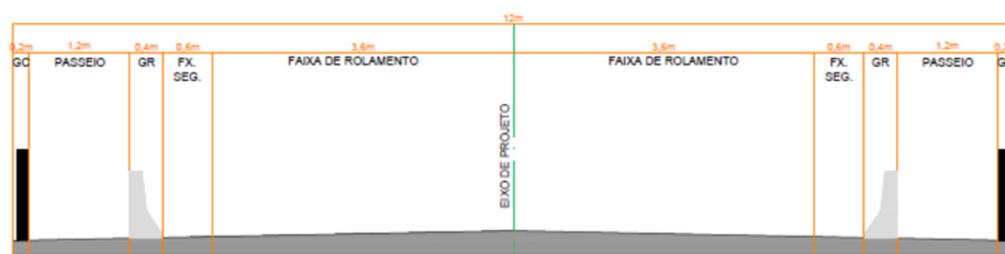
Figura 17: Dimensionamento da ponte
